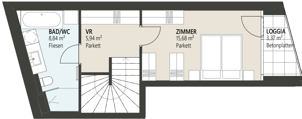
1. OBERGESCHOSS
