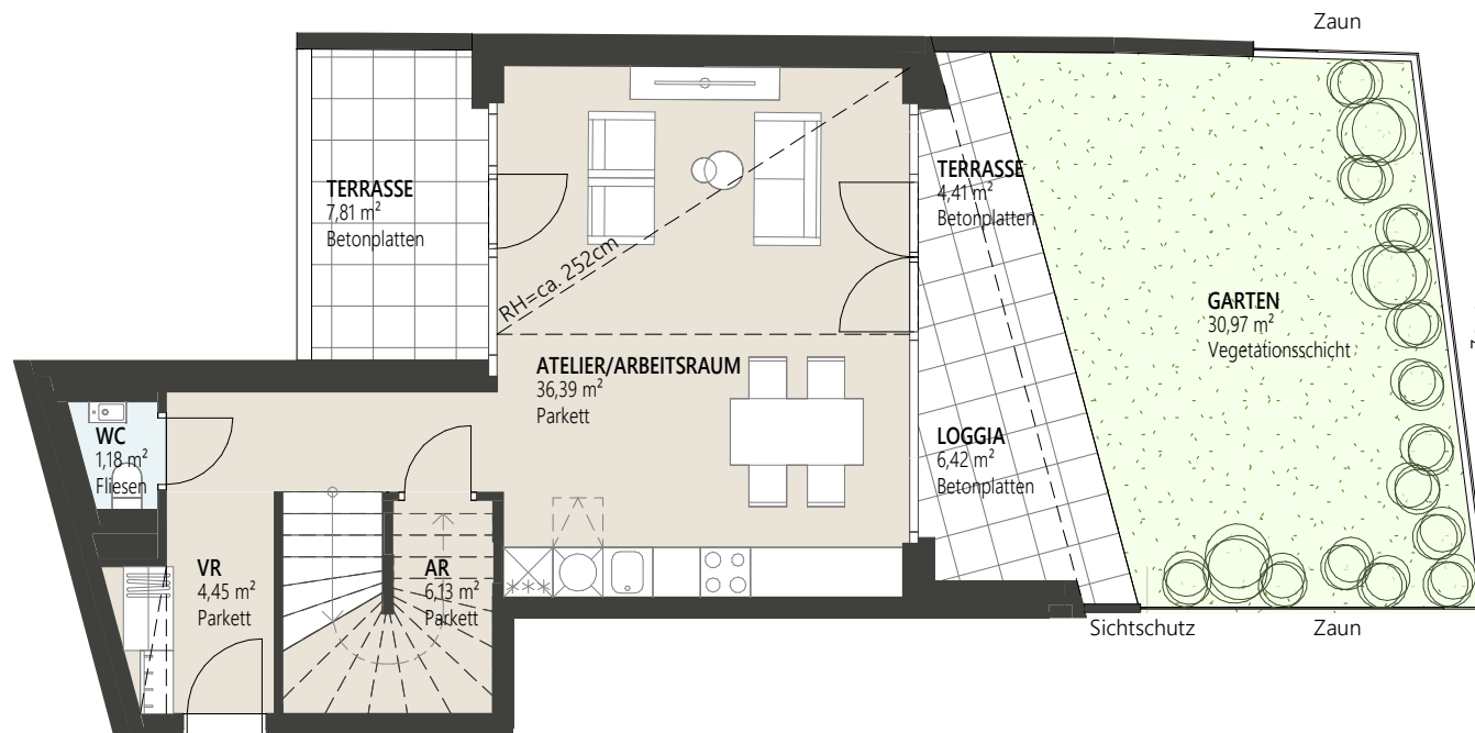
1. OBERGESCHOSS
