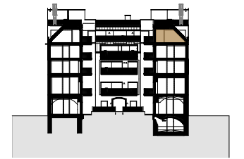
SCHNITT 3-3
