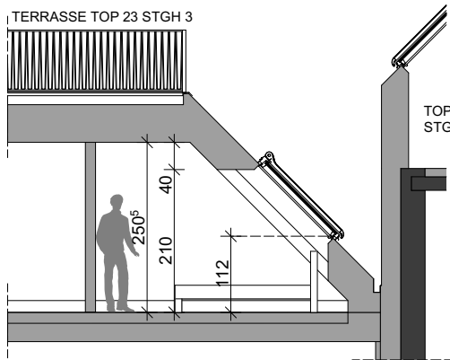
SCHNITT 2-2
