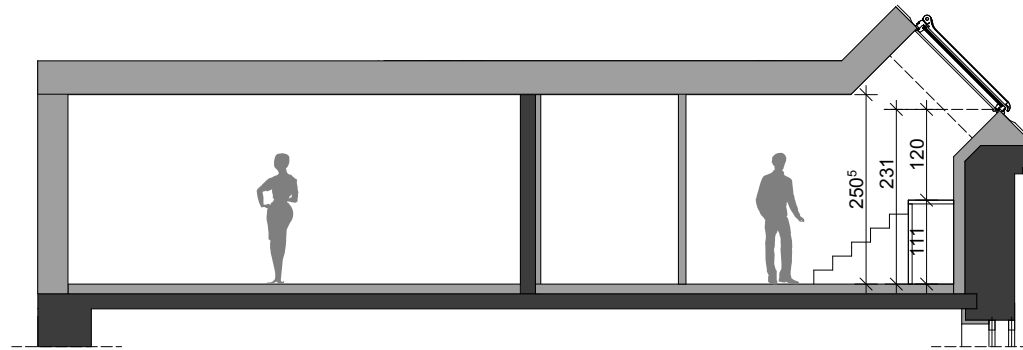
SCHNITT 3-3
