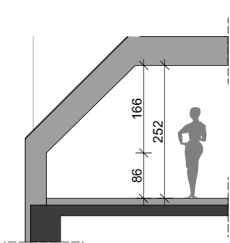
SCHNITT 2-2
