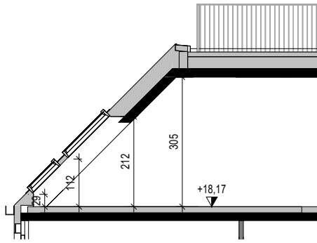
Schnitt 31.A
