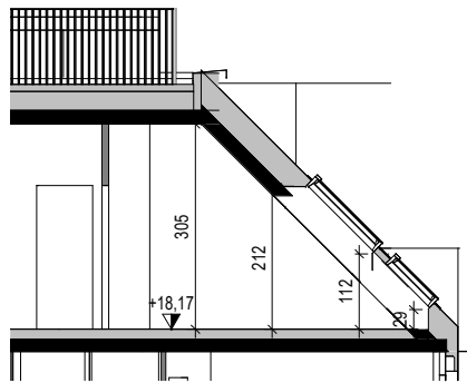
Schnitt 31.B
