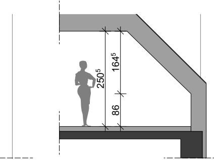
SCHNITT 2-2
