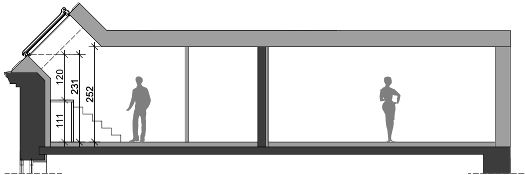
SCHNITT 3-3
